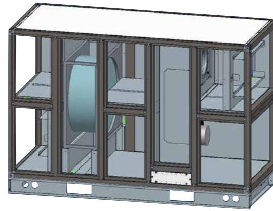
Recuperador rotativo con 100% aire exterior
