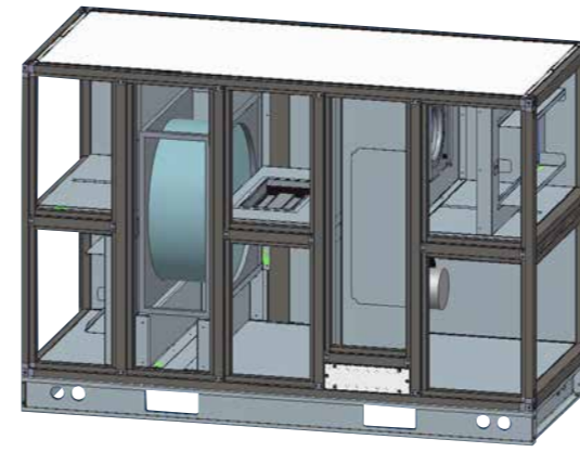
Recuperador rotativo con compuerta para recirculación de aire
