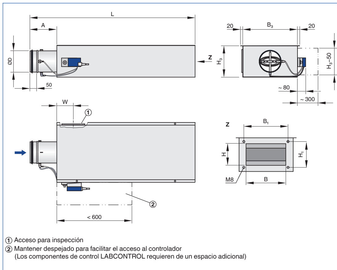
Croquis dimensional - detalle del perfil del conducto de aire
