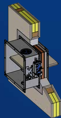
Instalación en pared estructural de madera
