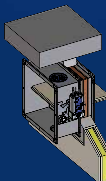
Distancia mínima a estructuras soporte (40 mm)
