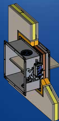
Instalación en panel de lana mineral resistente al fuego
