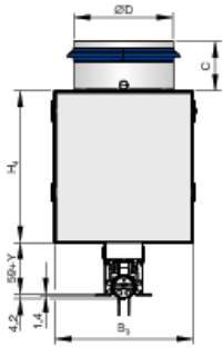
Tramo en esquina PL50-*-CS
