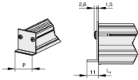
Remate en ángulo para perfil frontal del difusor con B00
