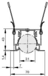
PL50-2-*.DF-*.B00 (perfil frontal con muelles)
