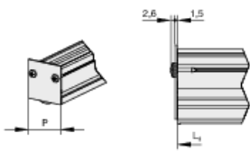
Remate final plano para perfil frontal del difusor con B00
