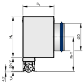
PL50*-PF-VS (plenum simétrico con boca para conexión vertical)
