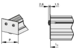
Remate en ángulo para perfil frontal del difusor sin B00
