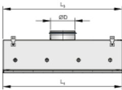
Puntos para fijación del plenum
