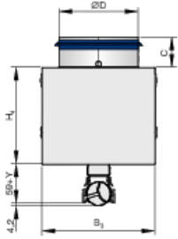
PL50-*-SF-VS (plenum simétrico con boca vertical)
