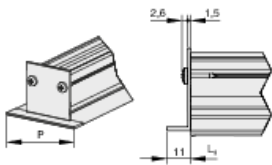
Remate en ángulo para perfil frontal del difusor con B00
