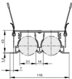
PL50-3-*.DF-*.B00 (perfil frontal con muelles)
