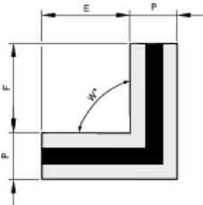
Remate plano EP para perfil frontal del difusor sin B00
