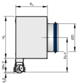
PL50*-SF-HA (plenum asimétrico con boca horizontal)
