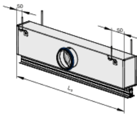
Disposición de la boca
