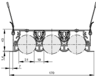
PL50-4-*.DF-*.B00 (perfil frontal con muelles)
