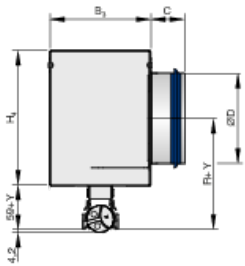
PL50*-SF-HS (plenum simétrico con boca horizontal)
