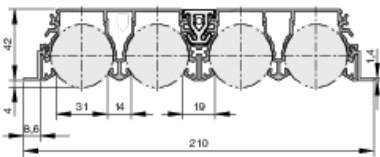
PL50-1-*.DF-*.B00 (perfil frontal con muelles)
