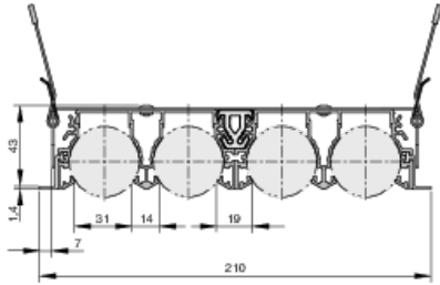
Plenum con boca horizontal (HS / HA)
